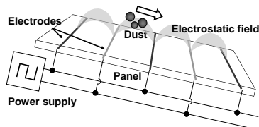
図 2 クリーナー概略図
