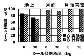
図 9 月面での性能の予測
