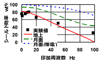
図 7 印加周波数特性
