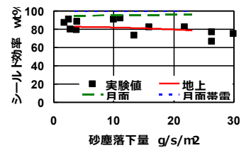
図 8 砂塵落下量特性 (計算)
